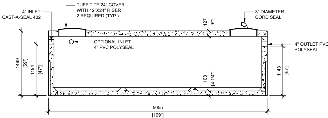
SECTION A SCALE: 1/50
