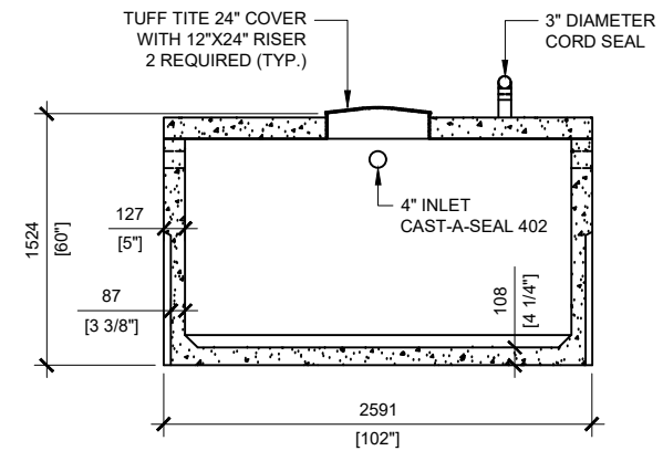
SECTION B SCALE: 1/50
