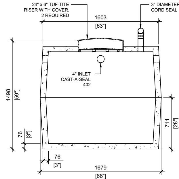
SECTION B SCALE: 1/30
