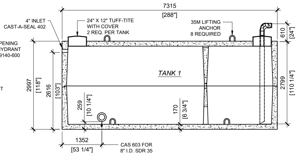
SECTION A SCALE: 1/80
