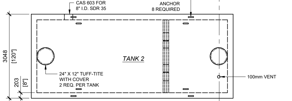
TOP VIEW SCALE: 1/80
