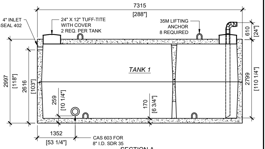
SECTION A SCALE: 1/80
