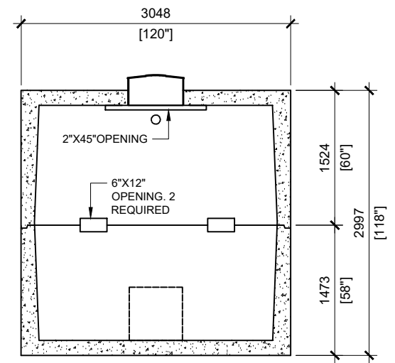
SECTION B SCALE: 1/60
