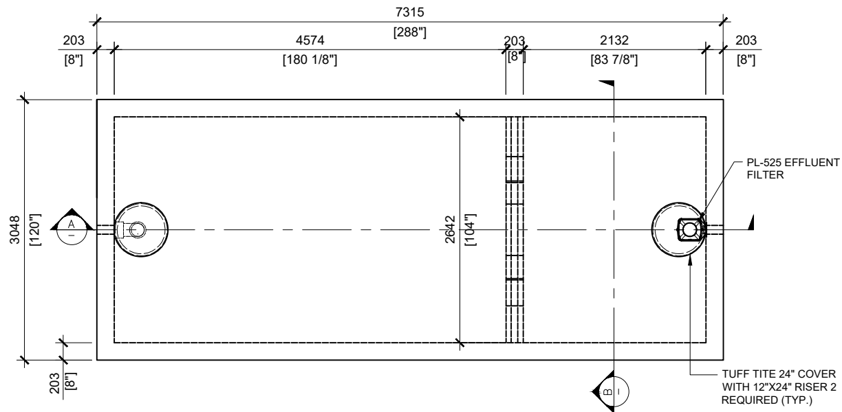
TOP VIEW SCALE: 1/60
