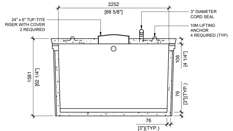
SECTION B SCALE: 1/40
