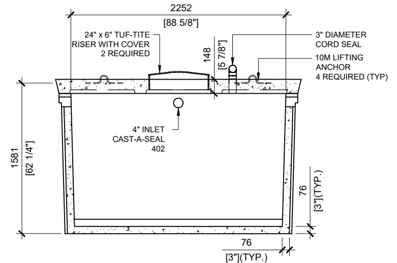
SECTION B SCALE: 1/40
