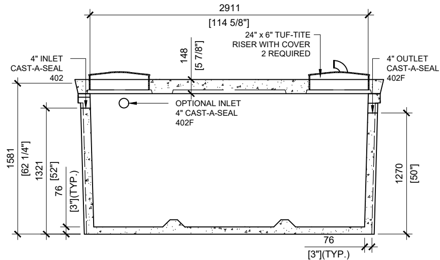
SECTION A SCALE: 1/40
