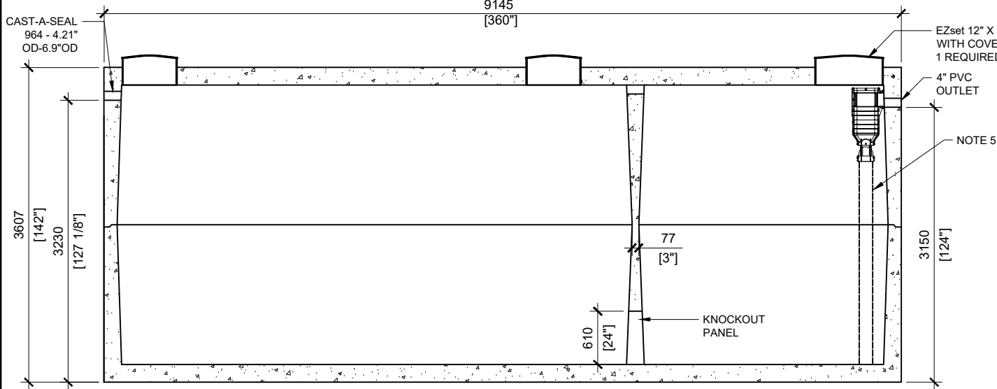
SECTION A SCALE: 1/30
