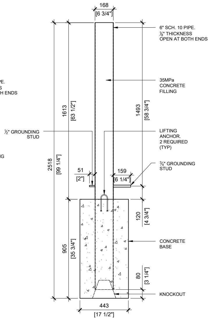
RIGHT VIEW SCALE: 1/20
