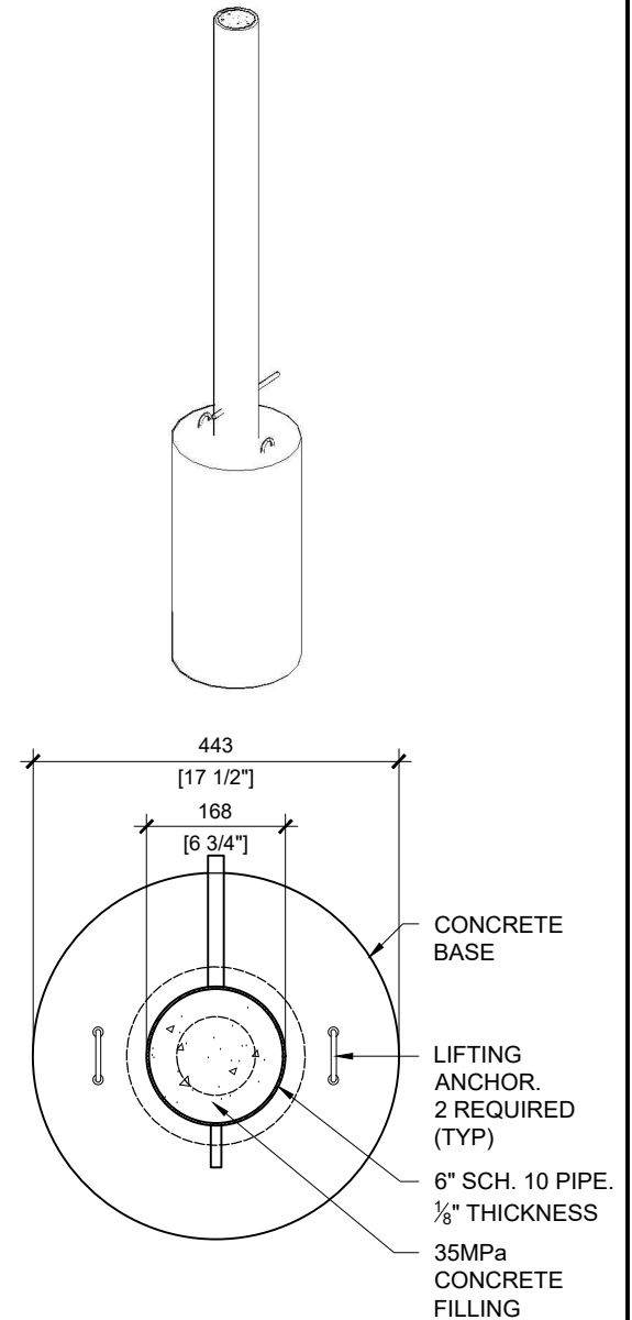
TOP VIEW SCALE: 1/10
