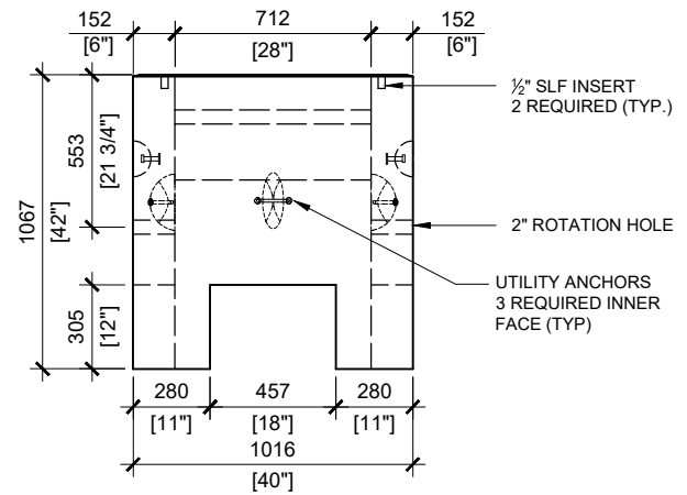
RIGHT VIEW SCALE: 1/30
