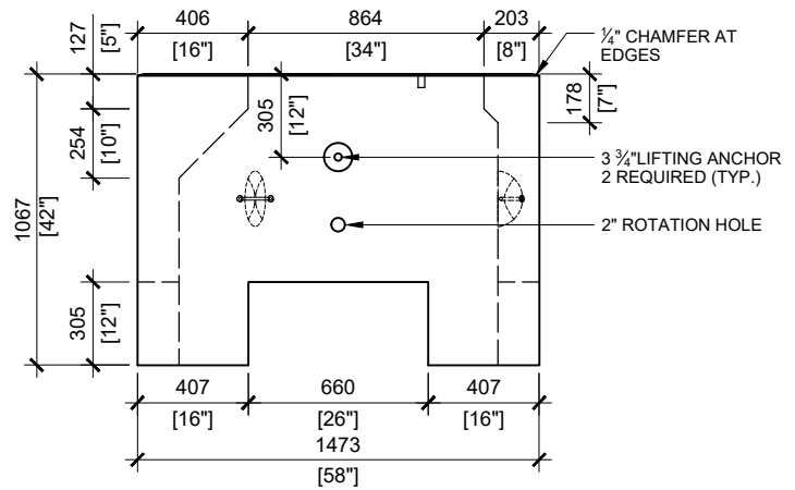
FRONT VIEW SCALE: 1:30
