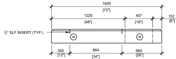
RIGHT VIEW SCALE: 1/30
