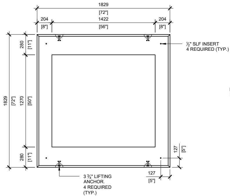
TOP VIEW SCALE: 1/30
