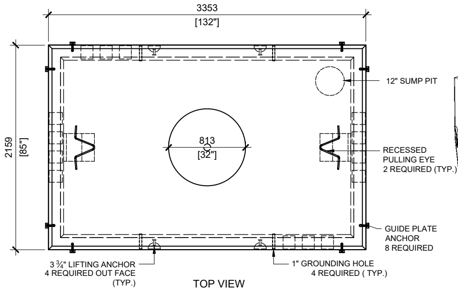
TOP VIEW SCALE: 1/40
