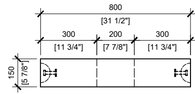
RIGHT VIEW SCALE: 1/20
