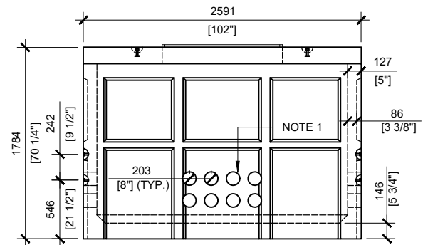
RIGHT VIEW SCALE: 1/50
