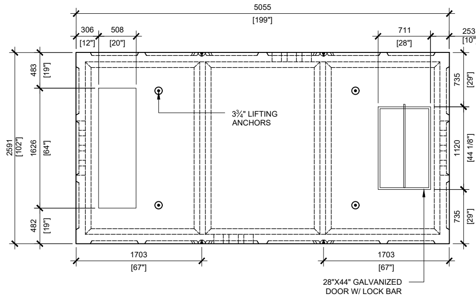
TOP VIEW SCALE: 1/50
