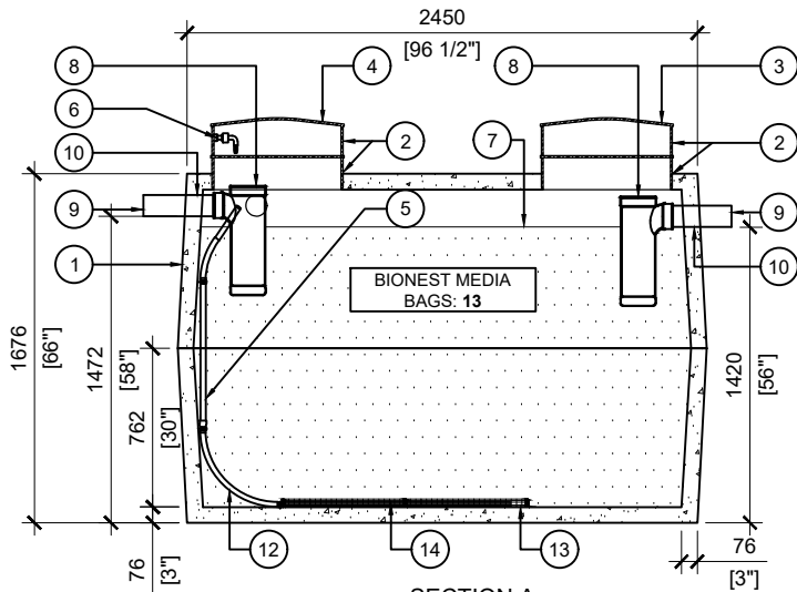
SECTION A SCALE: 1/30
