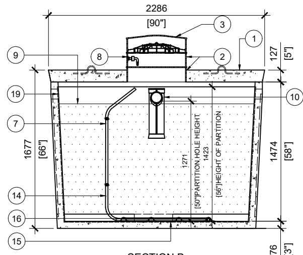
SECTION B SCALE: 1/40
