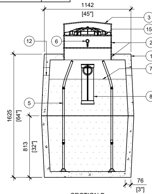
SECTION B SCALE: 1/30
