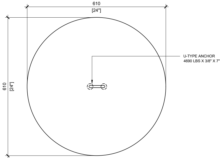
TOP VIEW SCALE: 1/8
