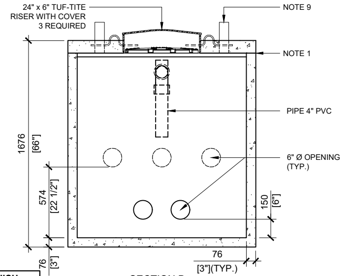
SECTION B SCALE: 1/30
