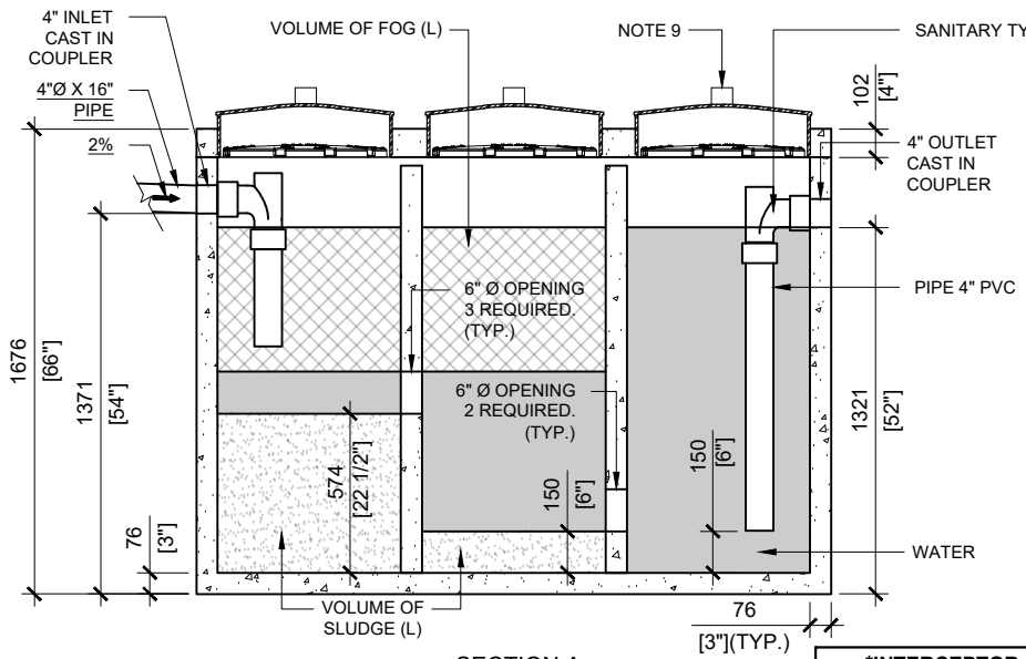
SECTION A SCALE: 1/30
