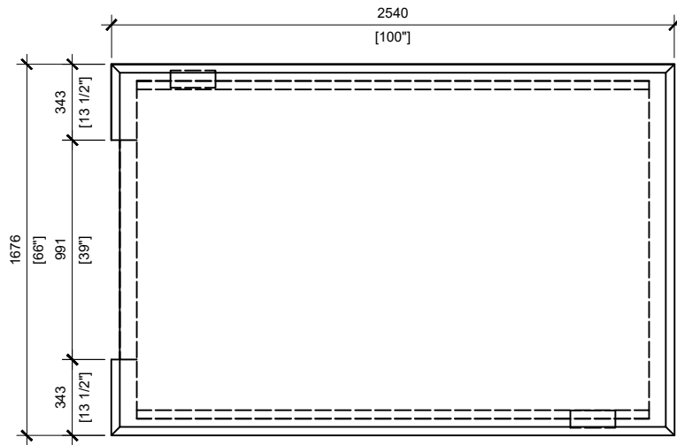
TOP VIEW SCALE: 1/30
