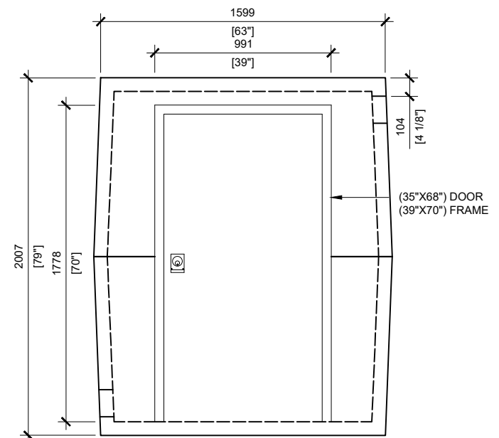
LEFT VIEW SCALE: 1/30
