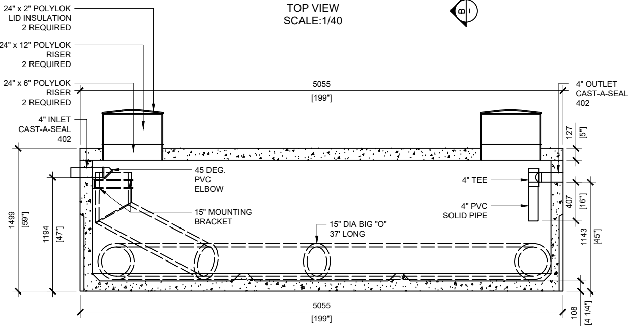
SECTION A SCALE: 1/40
