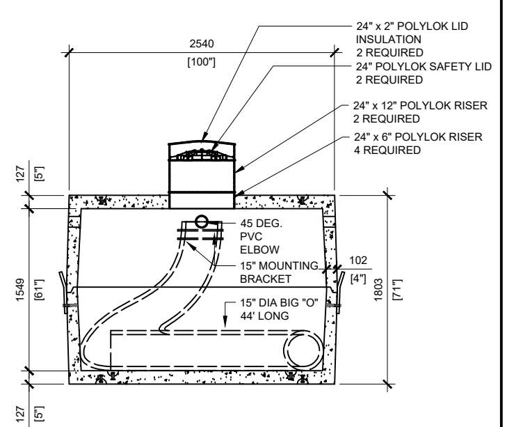
SECTION B SCALE: 1/50
