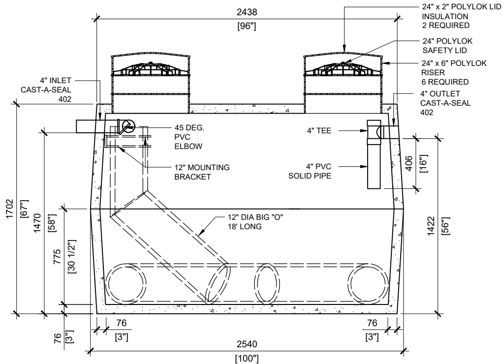
SECTION A SCALE: 1/30
