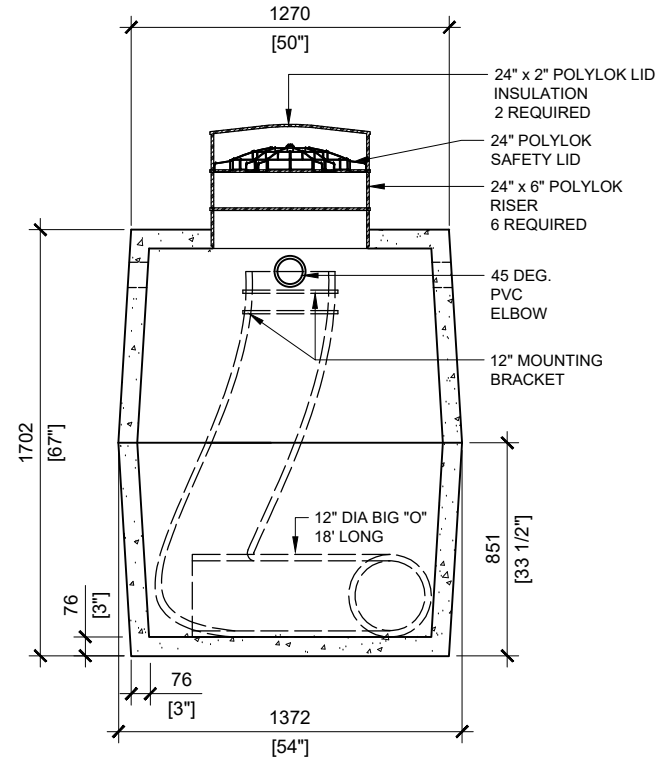
SECTION B SCALE: 1/30
