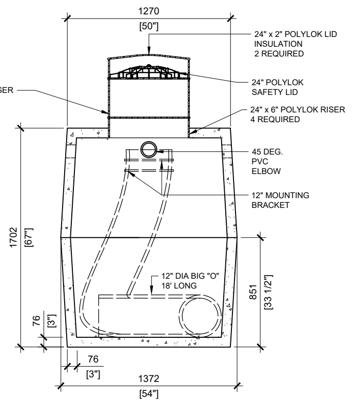
SECTION B SCALE: 1/30
