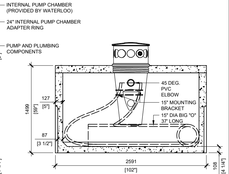
SECTION B SCALE: 1/40
