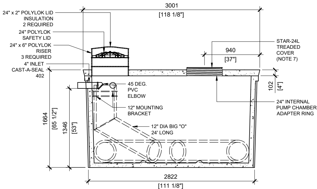
SECTION A SCALE: 1/40
