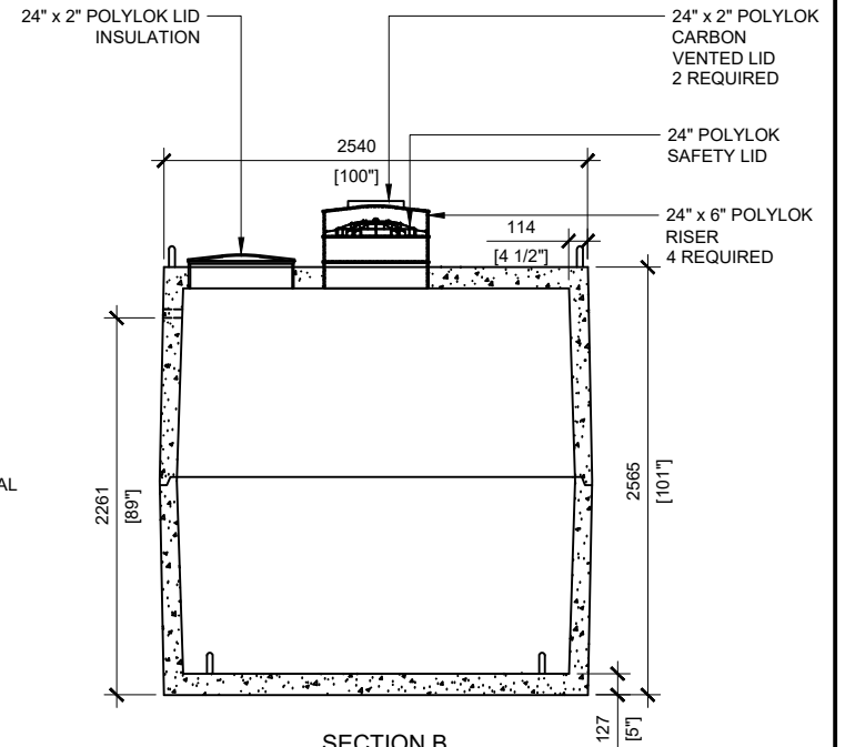
SECTION B SCALE: 1/50
