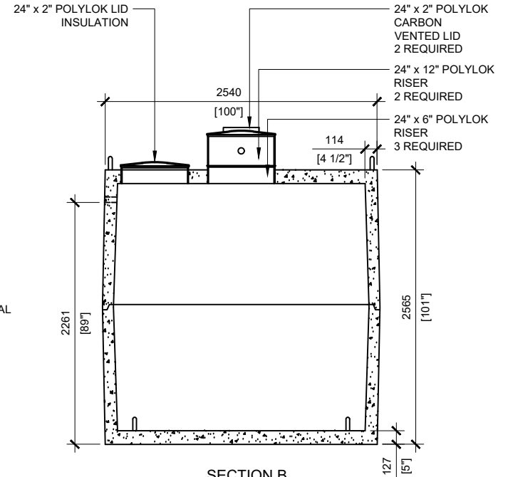
SECTION B SCALE: 1/50
