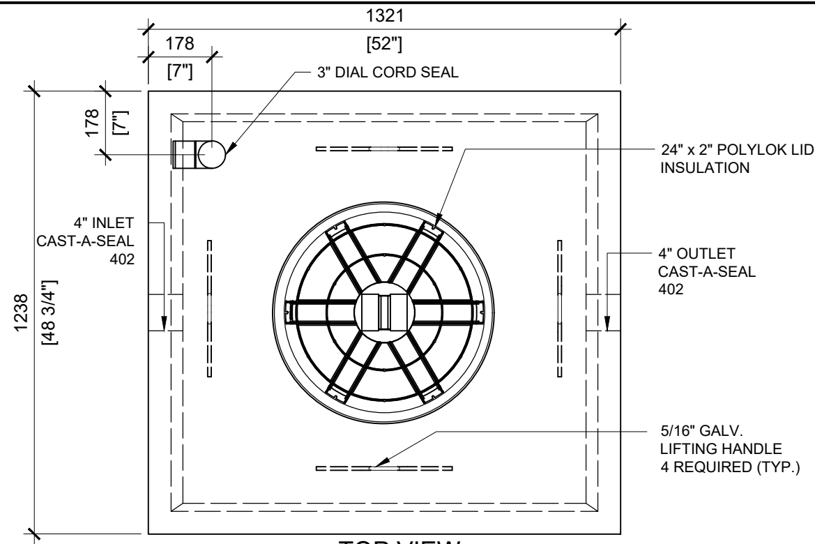
TOP VIEW SCALE: 1/20
