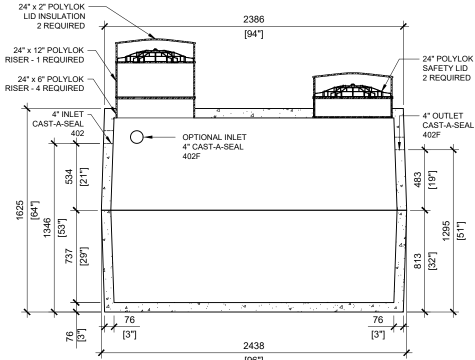
SECTION A SCALE: 1/30
