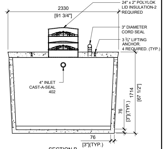
SECTION B SCALE: 1/40
