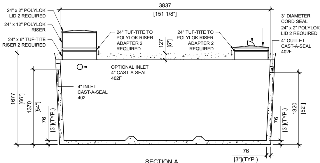
SECTION A SCALE: 1/40
