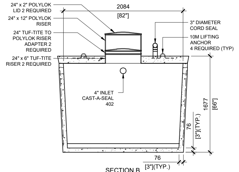
SECTION B SCALE: 1/40
