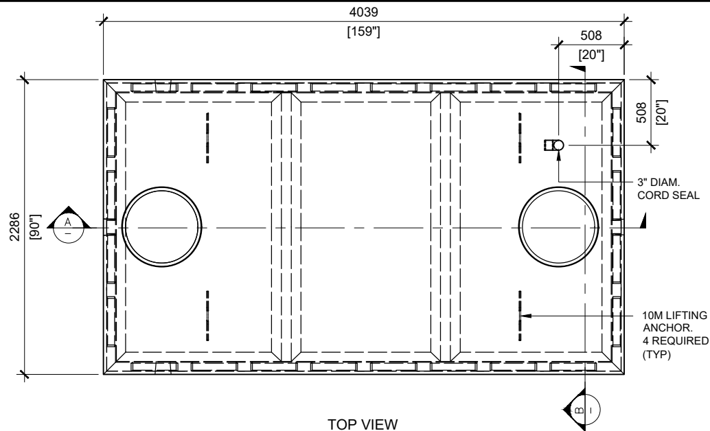
TOP VIEW SCALE: 1/40
