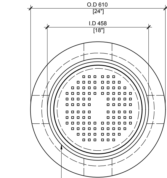
TOP VIEW SCALE: 1/10
