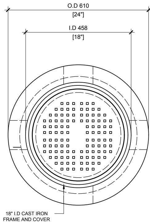
TOP VIEW SCALE: 1/10
